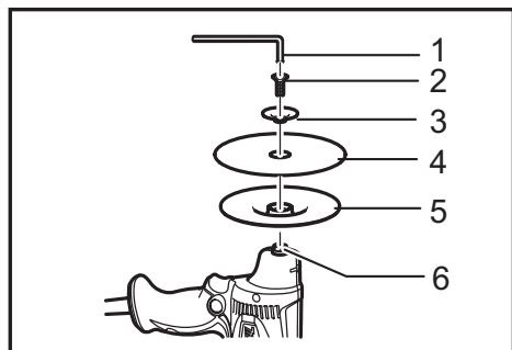
► 1. Clé hexagonale 2. Vis de serrage 3. Rondelle 4. Disque abrasif 5. Plateau en plastique 6. Axe
